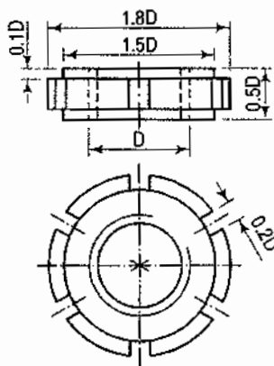
Ring nut
